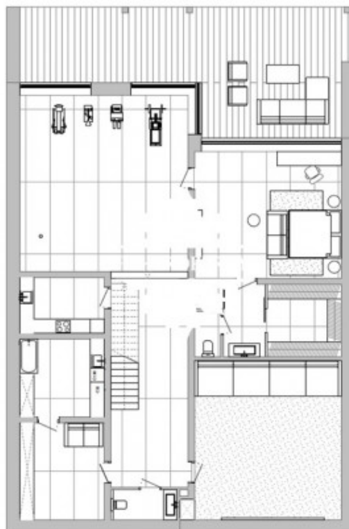
План с расстановкой мебели. Цокольный этаж
